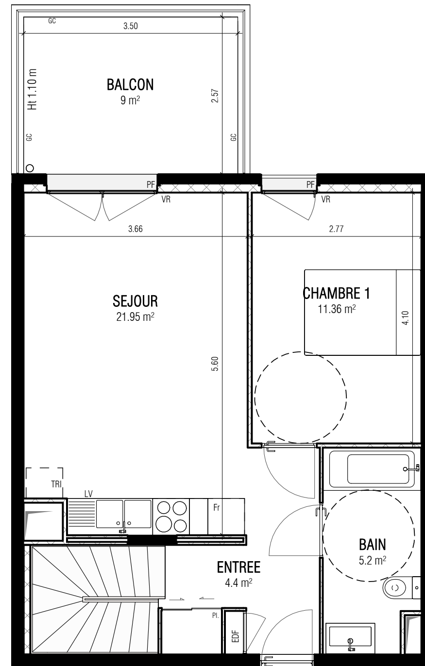
NIVEAU R+2
