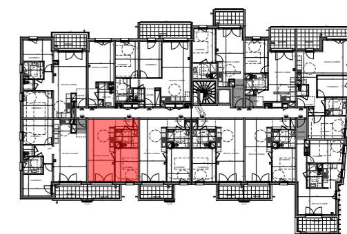
BÂTIMENT B Appartement de 2 pièces N°B-108 - 1er étage
