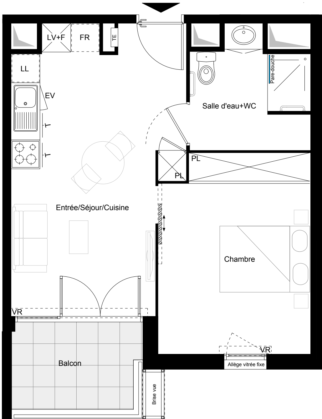
PLAN PROVISOIRE
