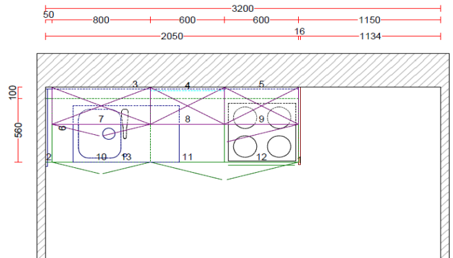
Plan d'élévation
